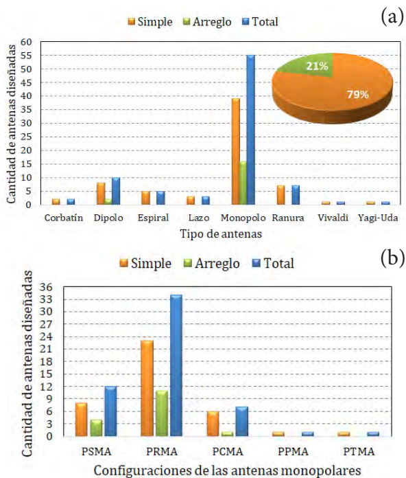
Figura 4. a) Antenas usadas en las rectenas y b) formas de parche de las antenas monopoles.
